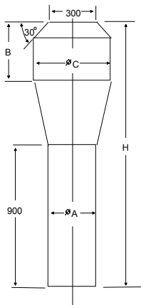
Mått: A = 300 mm., C = 450 mm., B = 300 mm., H = 1500 mm. Figur 2
